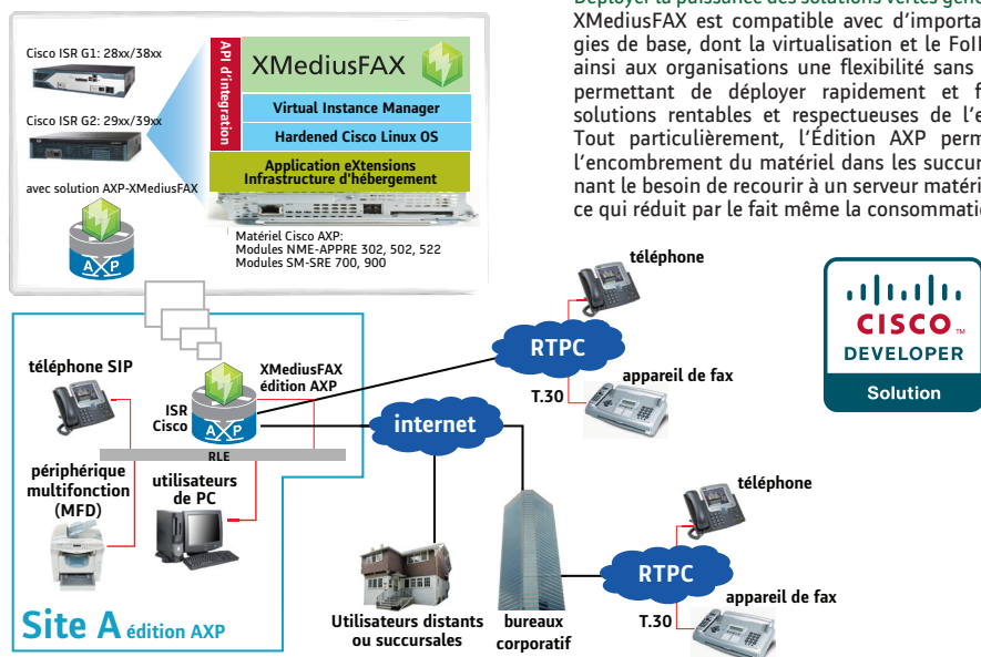
L'implantation typique de XMediusFAX Édition AXP dans une succursale
