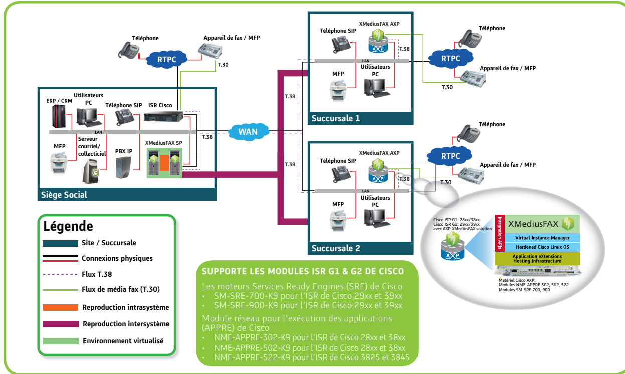
Figure 3 : XMediusFAX Édition AXP – architecture pour des succursales robustes aux pannes
