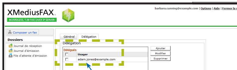
Figure 3 : Délégué ajouté
